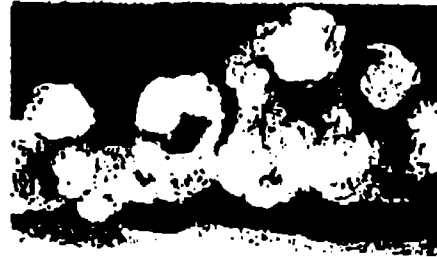
السحب ركامية ماطرة ضخمة
